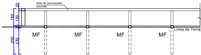
Elevação 02 esc.: 1/200
