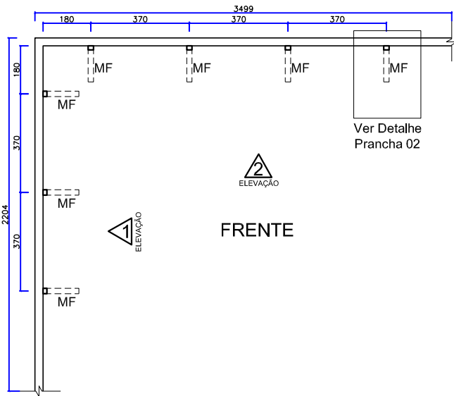
Planta de Localização das Estruturas - Frente esc.: 1/200
