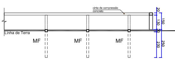
Elevação 01 esc.: 1/200
