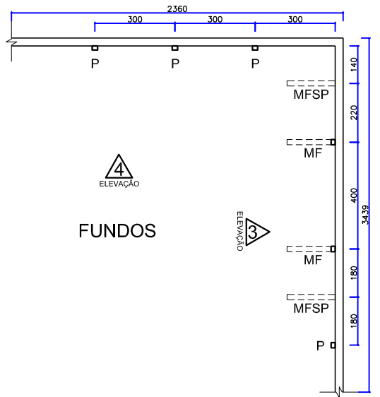
Planta de Localização das Estruturas - Fundos esc.: 1/200
