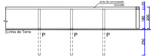
Elevação 04 esc.: 1/200
