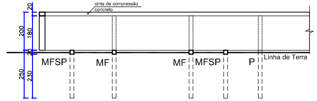
Elevação 03 esc.: 1/200
