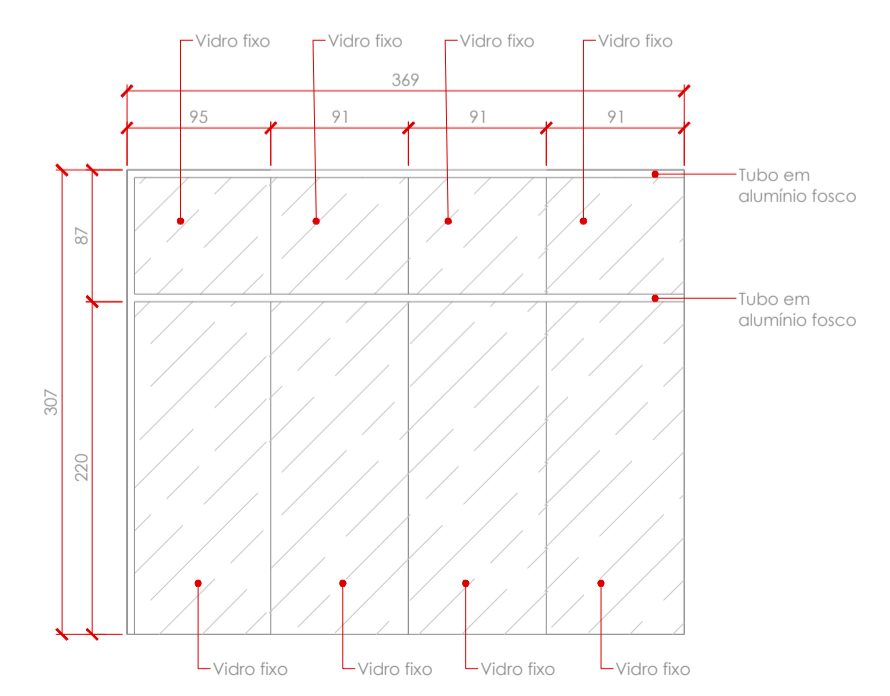
03 DETALHE 02 - PAREDE DE GESSO ESC.: 1/30
