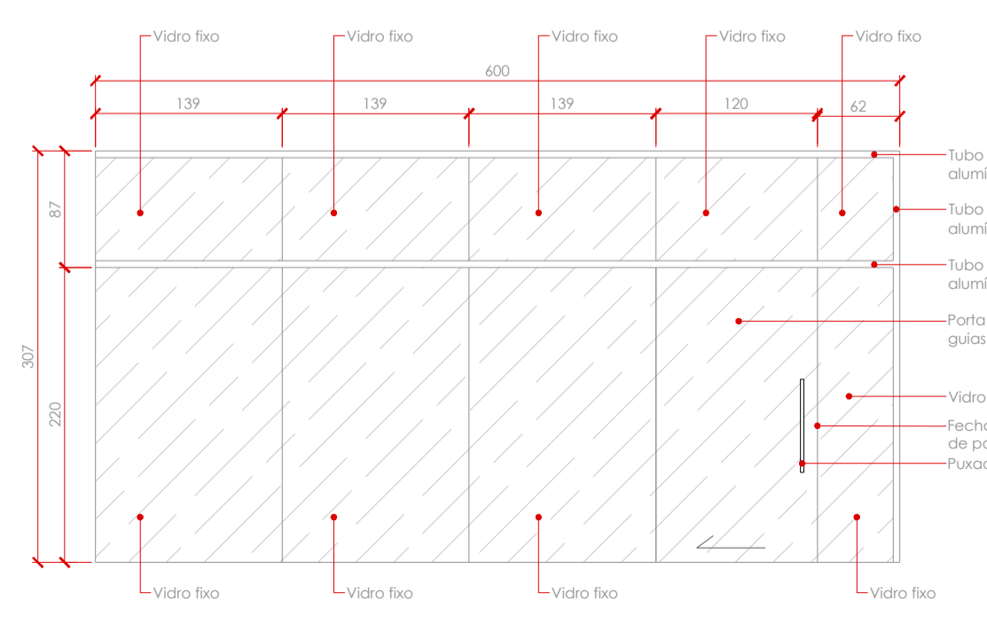
02 DETALHE 01 - PAREDE DE VIDRO ESC.: 1/30
