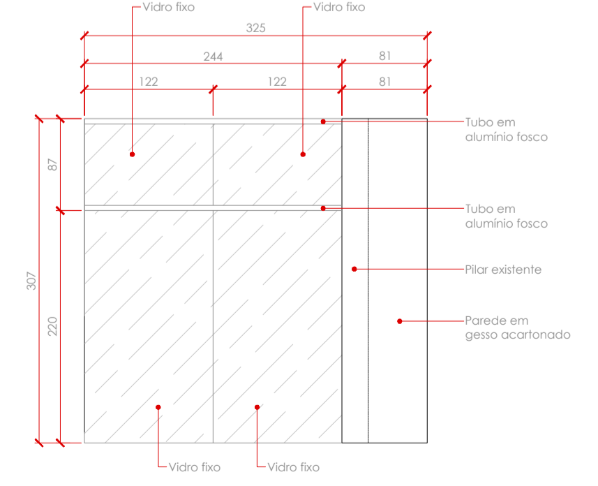
04 DETALHE 03 - PAREDE DE GESSO ACARTONADO E VIDRO ESC.: 1/30
