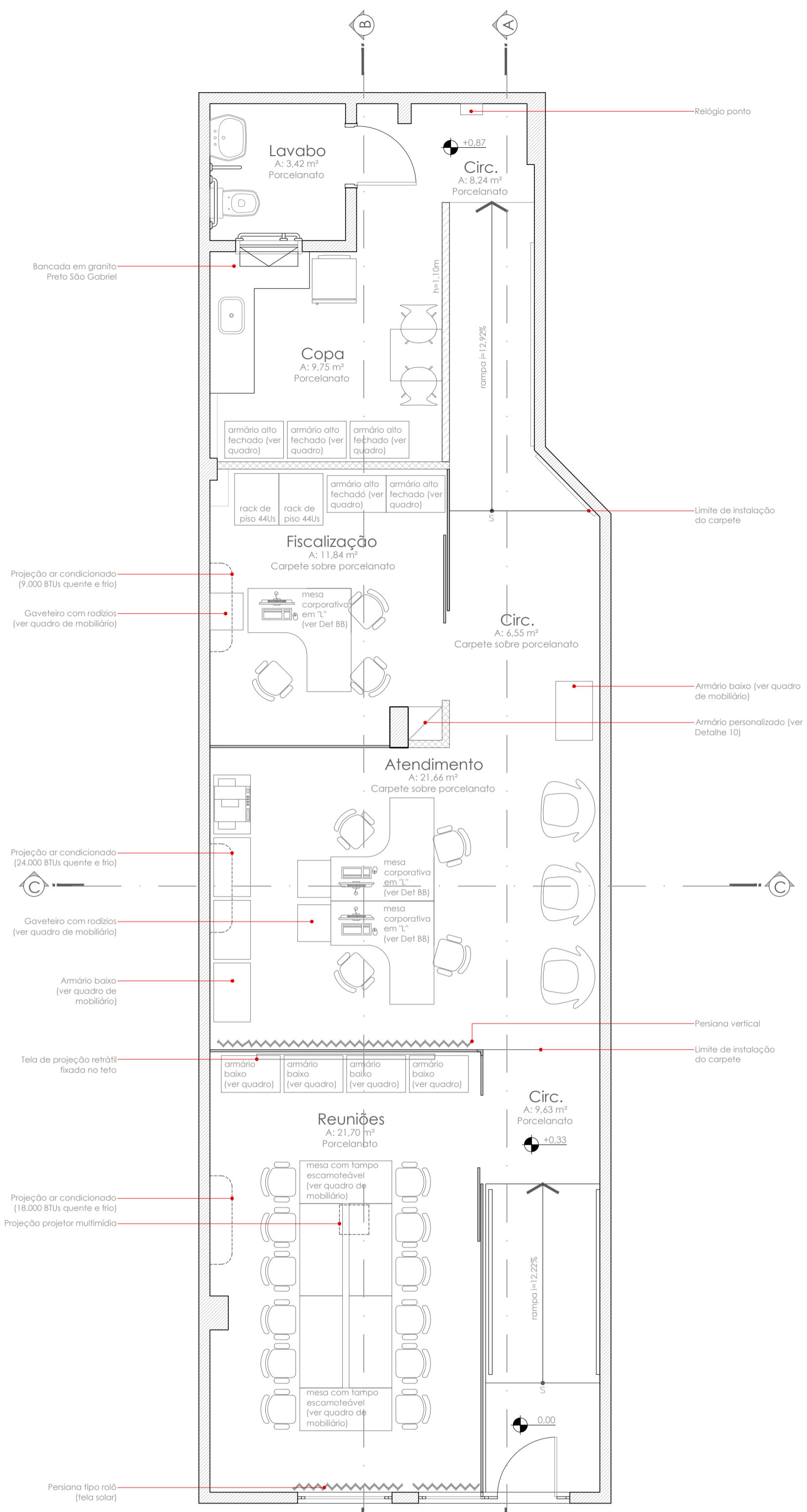
06 PLANTA BAIXA - LAYOUT ESC.: 1/50
