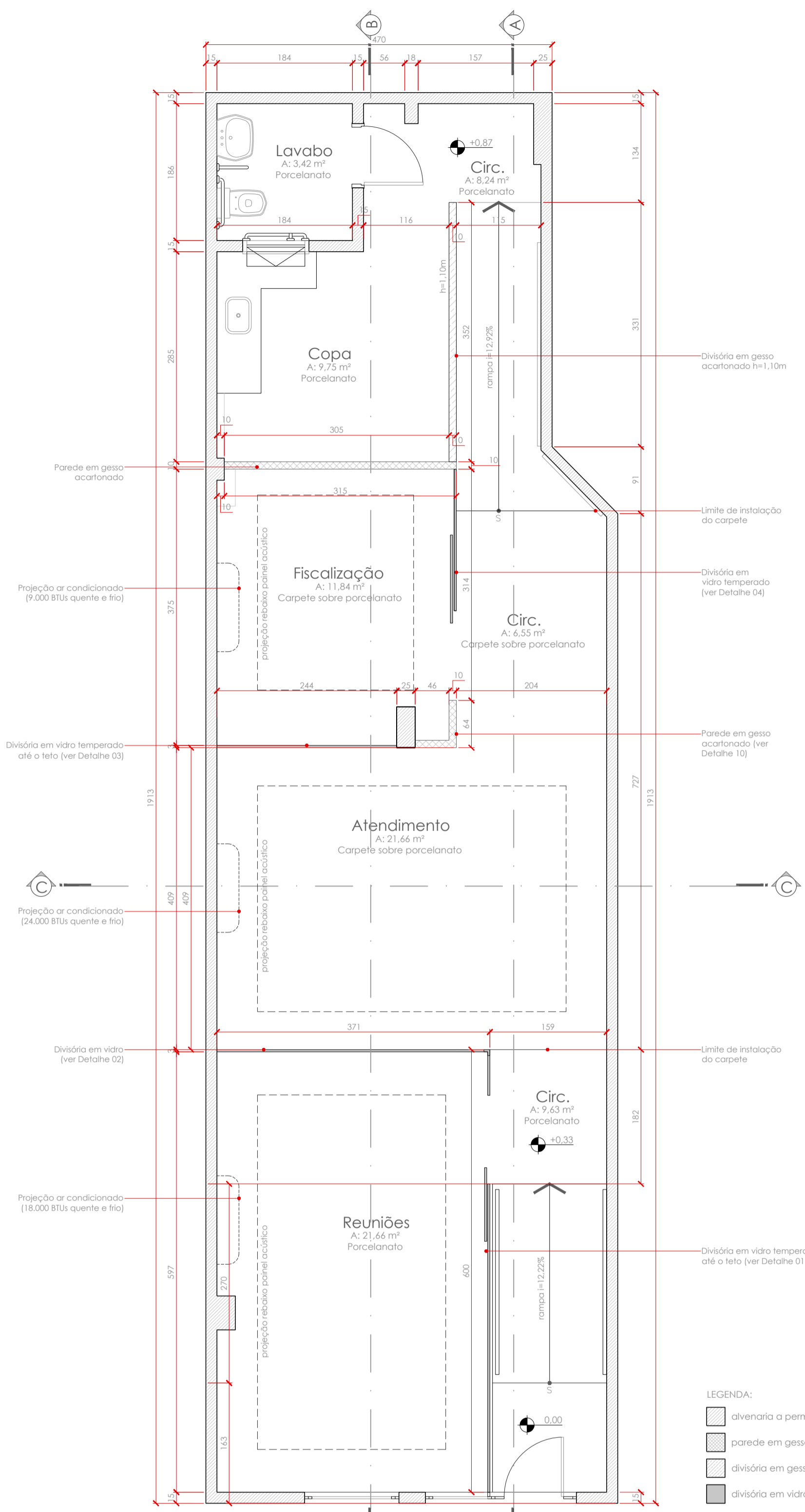
01 PLANTA BAIXA ESC.: 1/50
