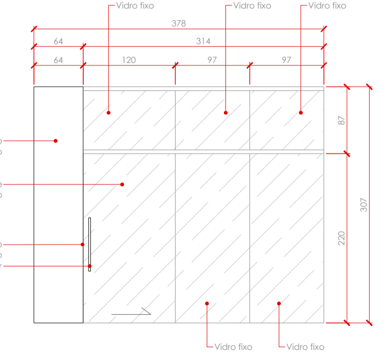
05 DETALHE 04 - PAREDE DE GESSO ACARTONADO E VIDRO ESC.: 1/30
